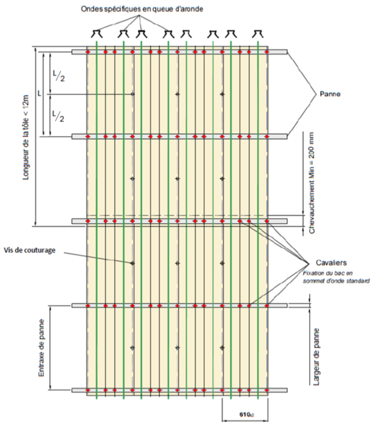
Figure 11 – Positionnement des fixations des plaques SOLABAC
