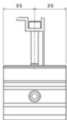
Figure 15 – Mise en place des modules et serrage des parcloses
