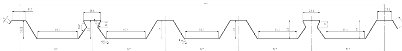
Figure 3 – Profil géométrique des plaques d'acier nervurées SOLABAC
