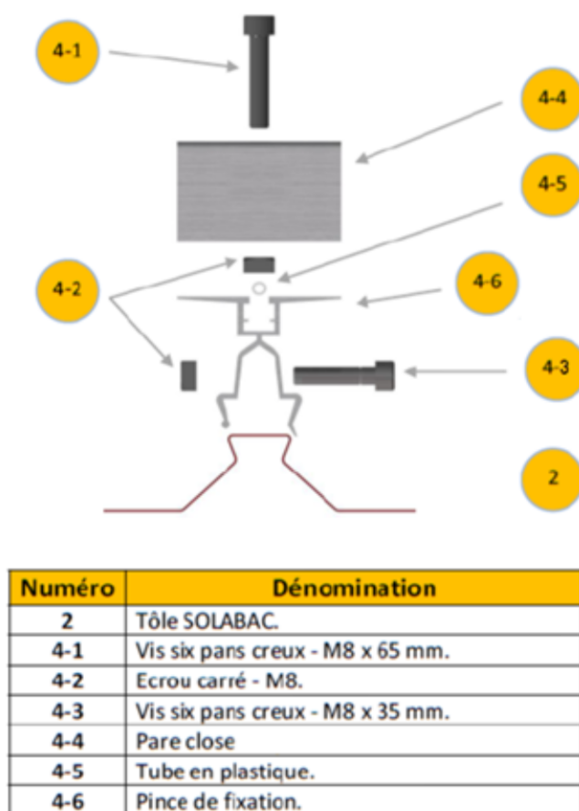
Figure 12 – Principe d'assemblage des pinces de fixation
