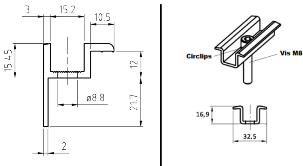
Figure 7 – Schémas des parcloles simple (à gauche) et double (à droite)
