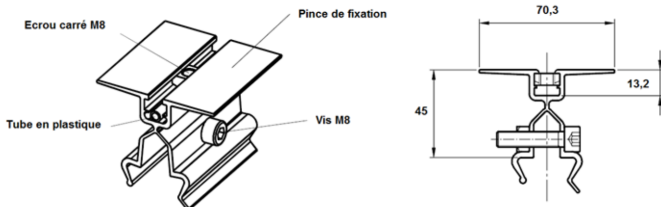
Figure 6 – Schémas des pinces de fixation
