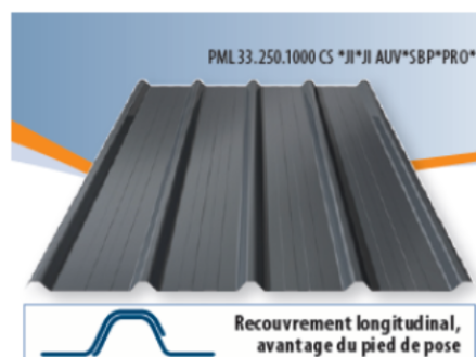
Figure 5 – Profil géométrique des plaques d'acier nervurées JORISIDE pour couverture partielle
