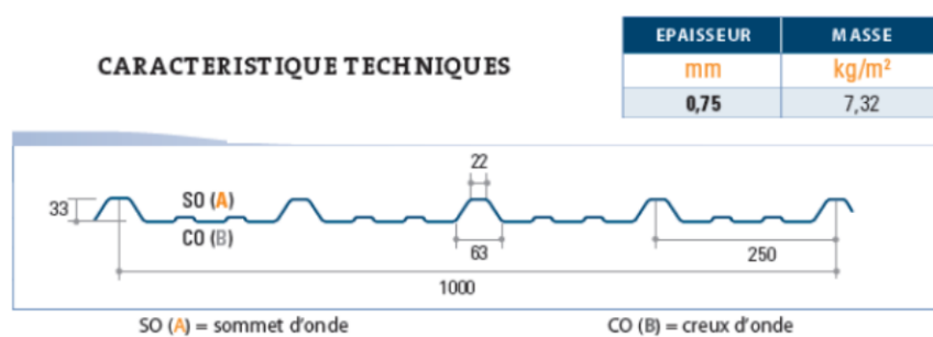
Figure 5 – Profil géométrique des plaques d'acier nervurées JORISIDE pour couverture partielle
