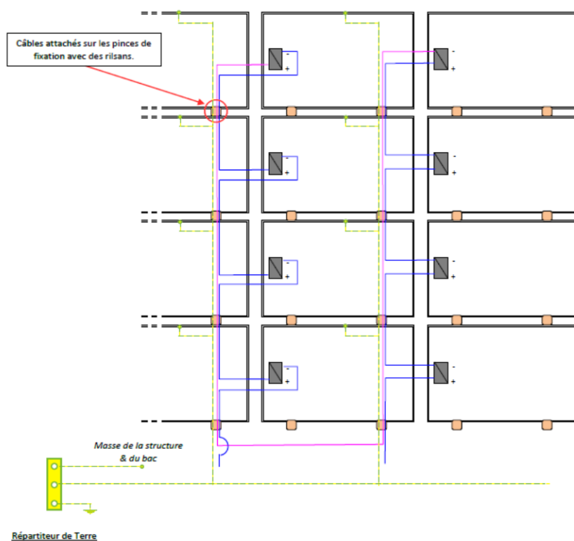
Figure 8 – Schéma de principe pour les liaisons électriques et liaisons équipotentielle des masses
