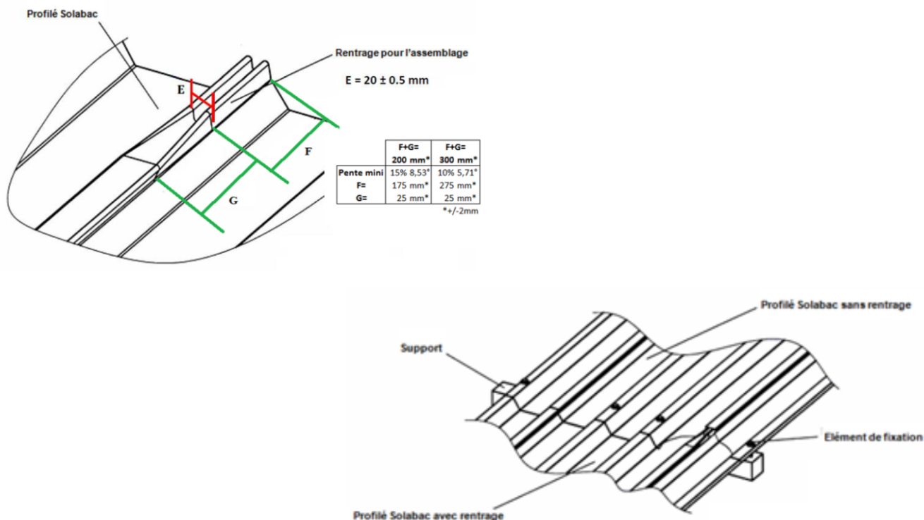
Figure 4 - Pliage en usine des nervures en queue d'aronde pour permettre le recouvrement transversal
