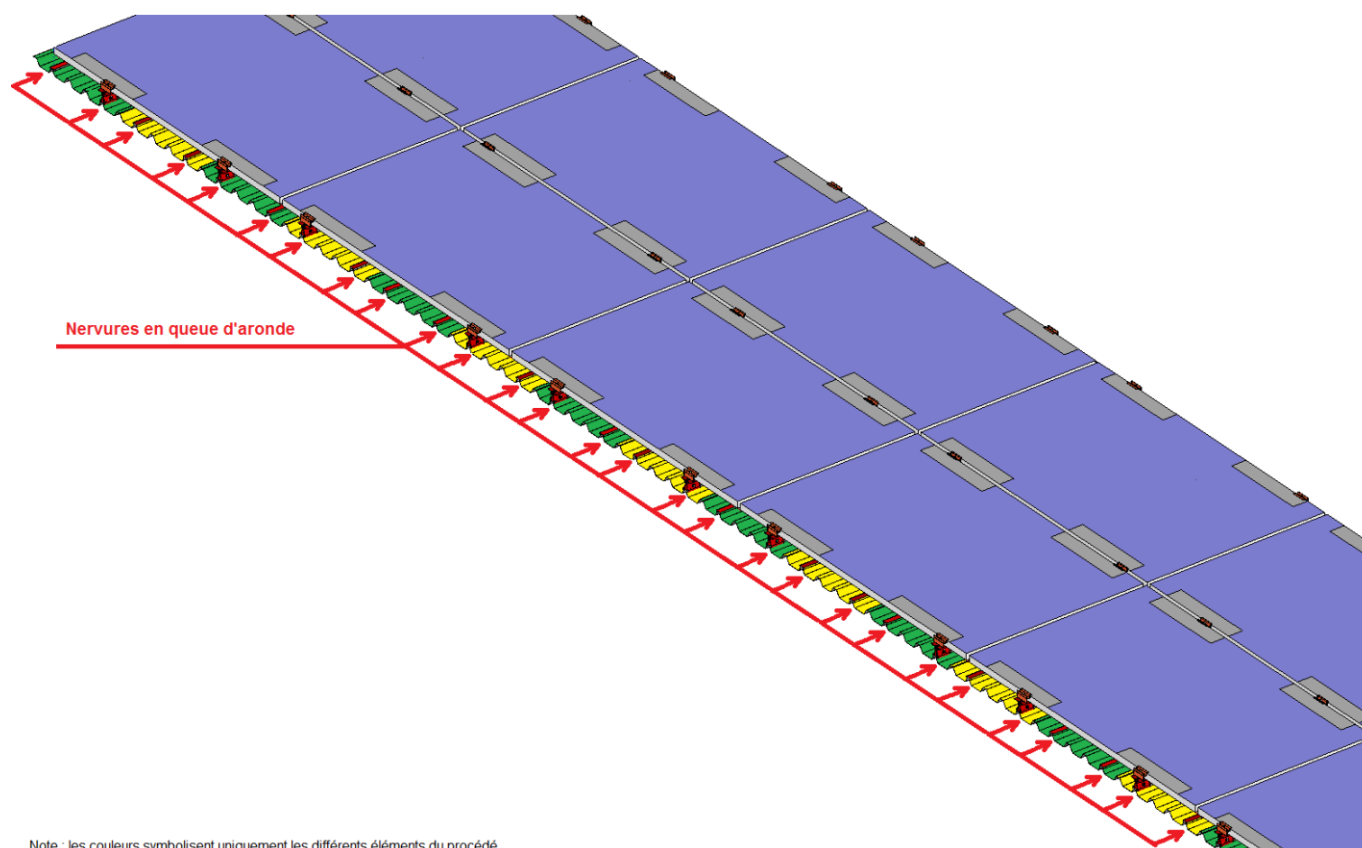
Figure 13 – Principe de calepinage des pinces sur les nervures en queue d'aronde
